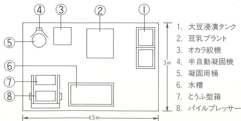
▲パイルプレッサー1060型
