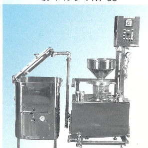
小型とうふプラント
