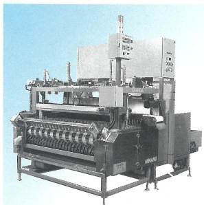
油揚、選別機エランダ
