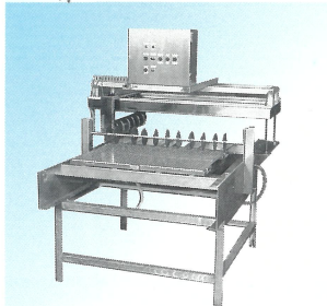
油揚、生地カッター
