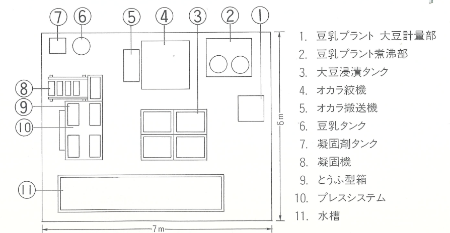
自動凝固システム、成型、プレス、カット▶
